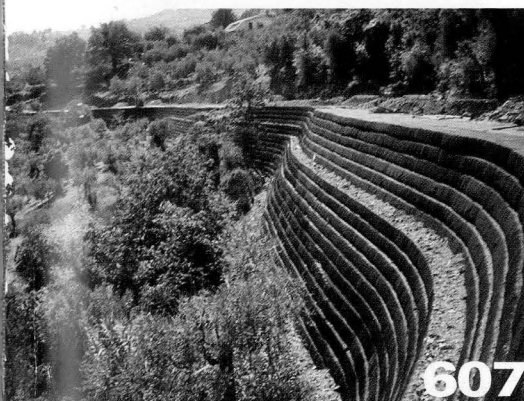
CONTENIMENTO TERRA
